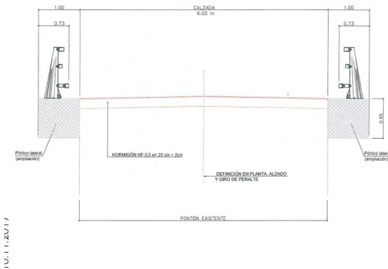
SECCIÓN TIPO PONTÓN 17-300 Escala 1:50
