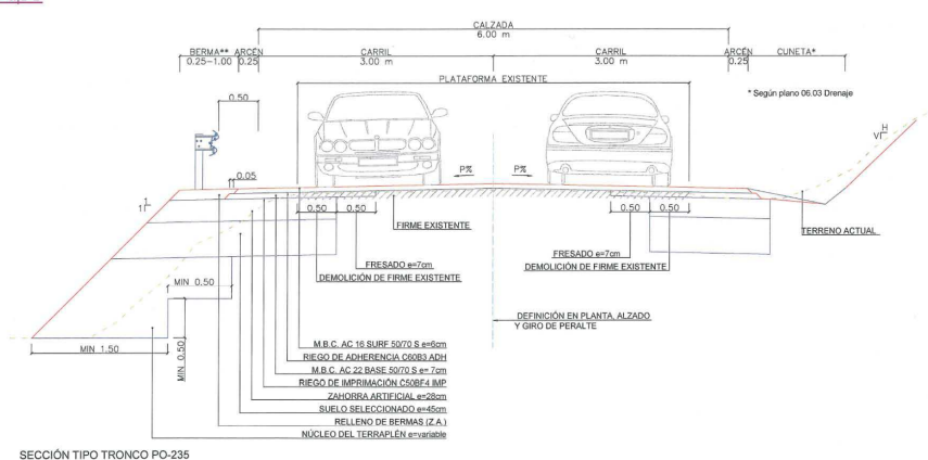
SECCIÓN TIPO TRONCO PO-235
