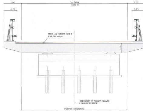
SECCIÓN TIPO PONTÓN 154-630 Escala 1:50
