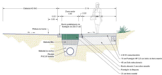
Sección tipo
