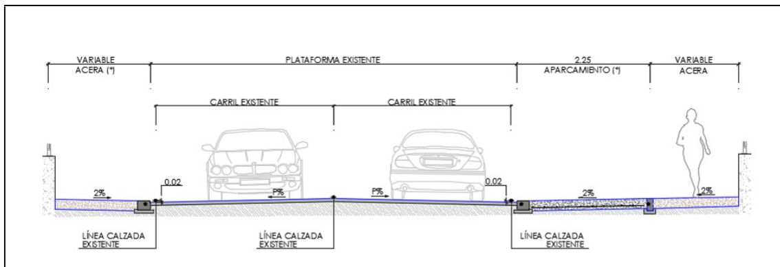
Sección tipo travesía de Liñares. Tramos de beirarrúa e aparcamento segundo tramos
